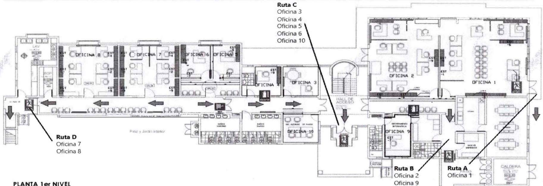
PLANTA 1er NIVEL esc. 1:50
