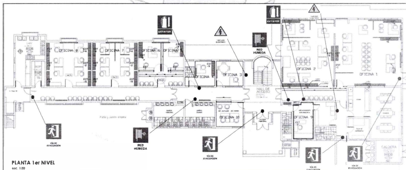
Figura 7 - Alarma y Recursos (primer nivel) Municipalidad Provisoria.
