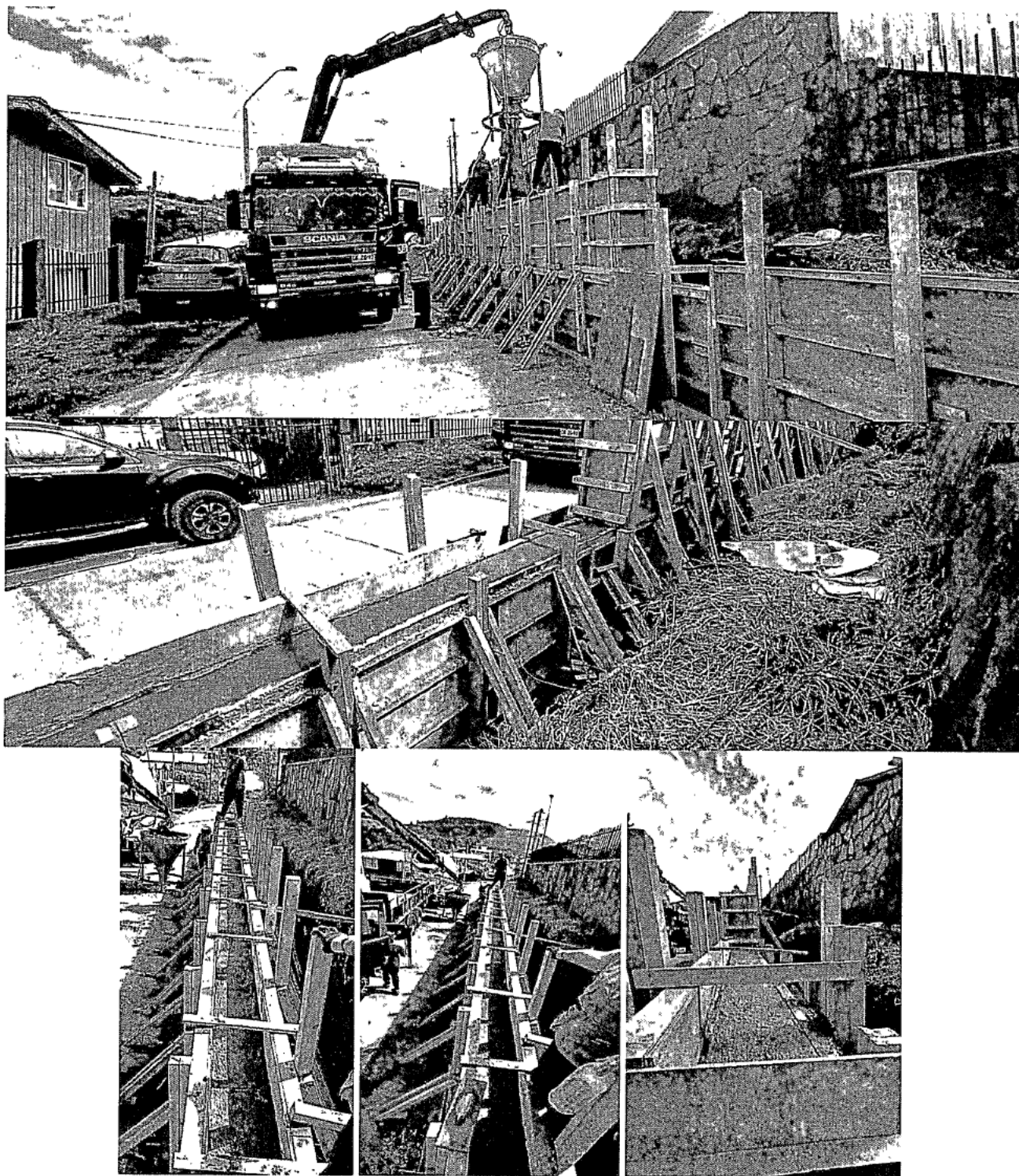
Imagen 4: Hormigonado de pantalla de muro en largo total de 18 m.
