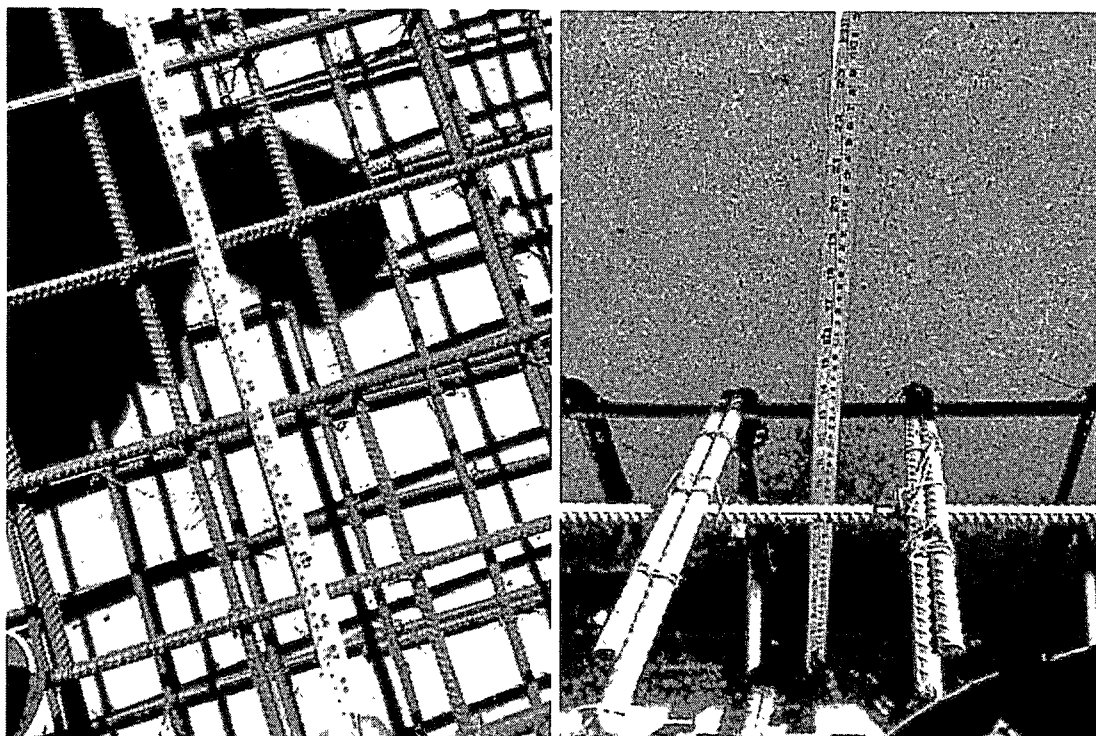
Foto 1: Control de distanciamiento entre perfiles cada 15 cm / Foto 2: Control de espesor de enfierradura de zapata de 35 cm, con recubrimiento de 2,5 cm por lado (altura total 40 cm).
