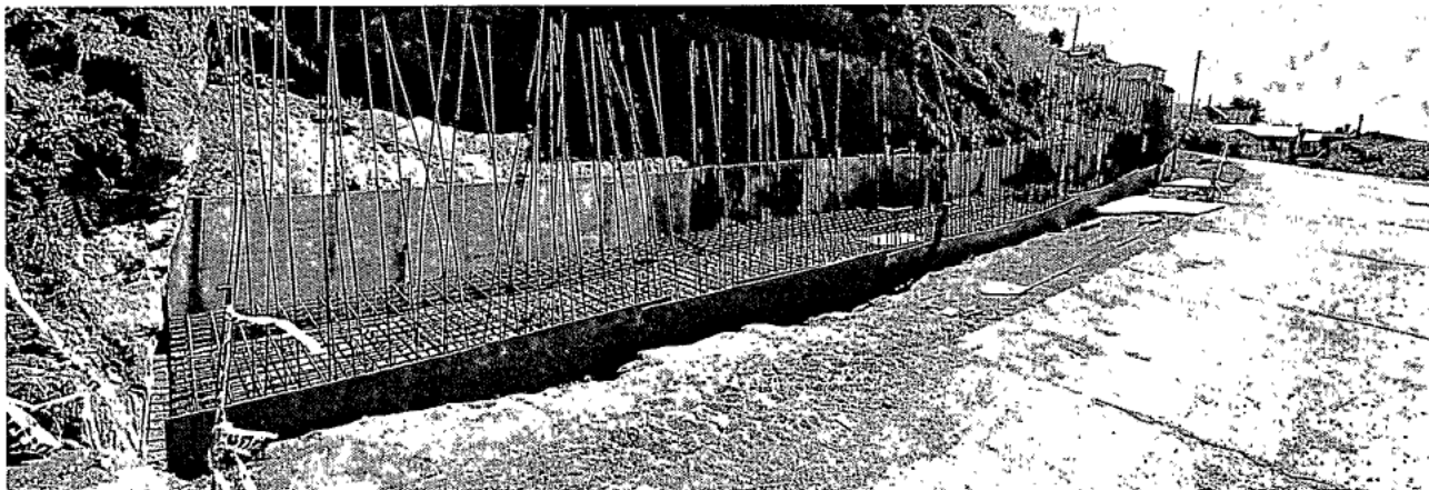
Imagen 5: Instalación de malla de zapata en perfiles fe12 y distanciamiento cada 15 cm.
