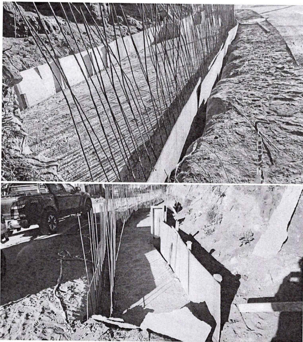
Imagen 6: Hormigonado de zapata de muro mediante hormigón de calidad H-30.
