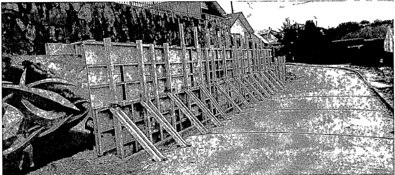
Imagen 3: Instalación de moldajes para pantalla de muro, con caras verticales aplomadas y recepcionadas.
