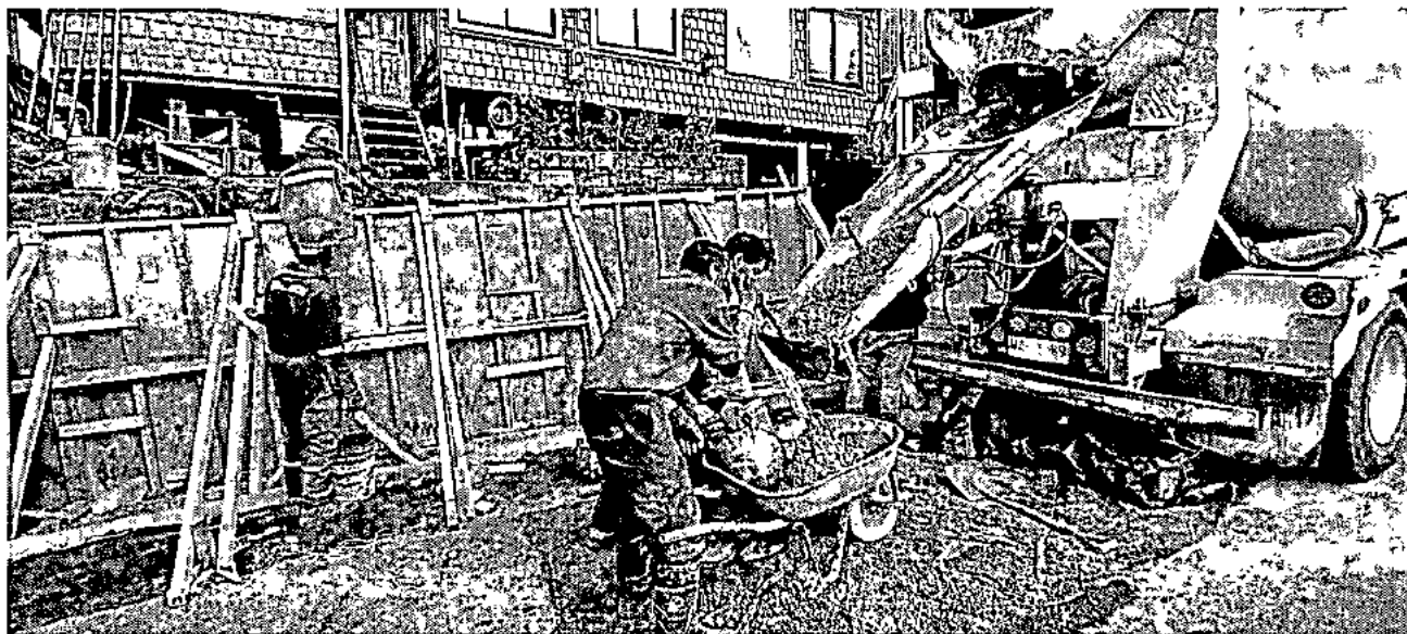
Imagen 11: Instalación de moldaje en pantalla de muro (9,2 ml).
