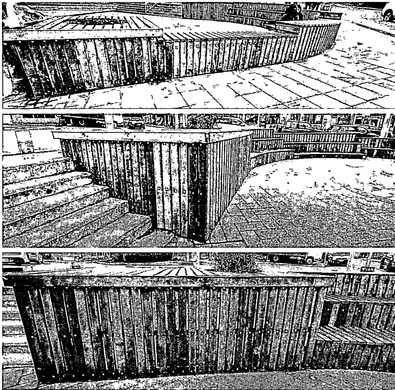
Imagen 1: Instalación total de entablado de pino 1x4" en cara horizontal y vertical para banca continua sobre estructura de fijación existente (reacondicionada).
