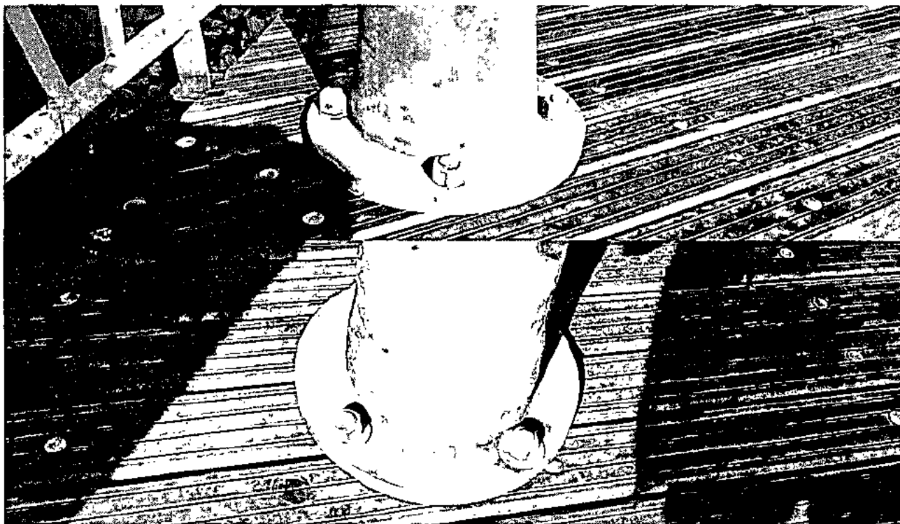
Imagen 4: Fijación de focos a entablado de piso; se aplica pintura antioxidante sobre pernos de fijación.
