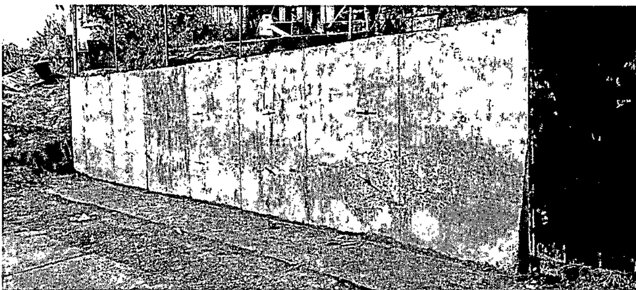
Imagen 12: Hormigonado de pantalla de muro en un largo total de 9,2 m y en calidad H-30.
