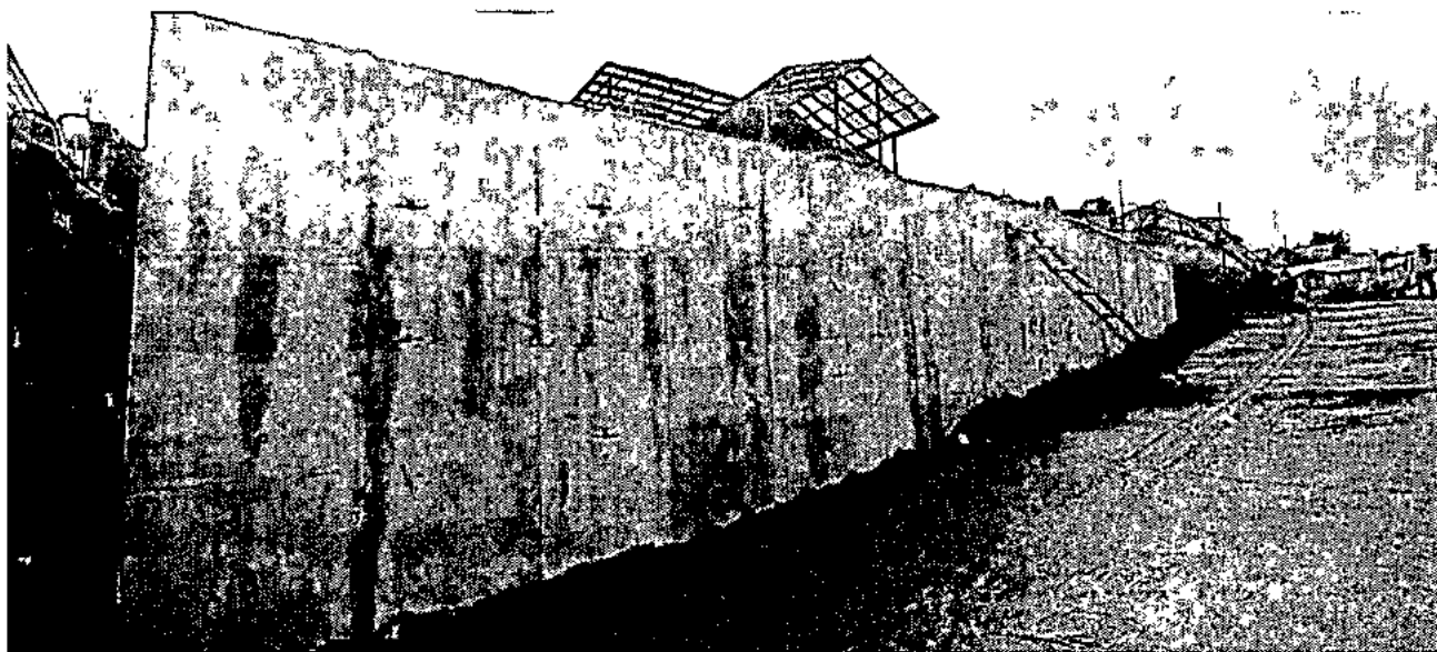
Imagen 9: Hormigonado de 25 m de pantalla de muro en hormigón de calidad H-30.
